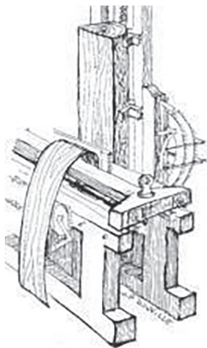
Scie au bois montant de M. Cochot (1799). Dessin Douville. Histoire du bois de placage.
